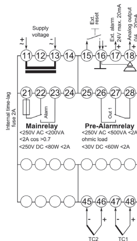
Thermocouple 2RAO
