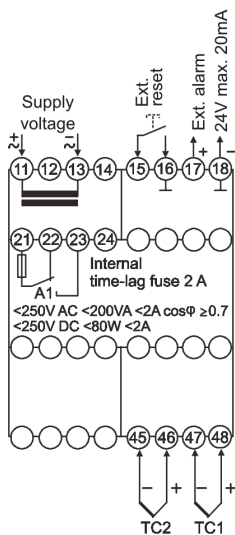
Thermocouple 1R
