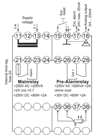
Pt100-2RAO
