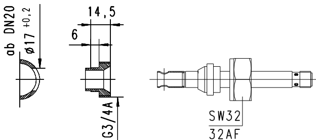
Einschweißadapter
