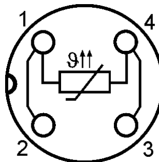
Anschlussvariante 2 (kundenspezifisch)
