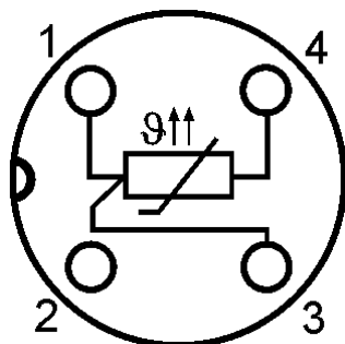
Anschlussvariante 1 (Standard)
