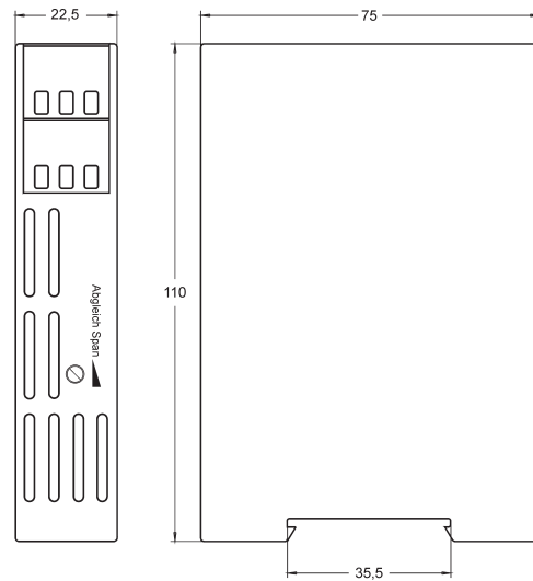
Tragschienenmontage TS35
